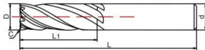
5-зубая концевая фреза для жаропрочных и титановых сплавов
